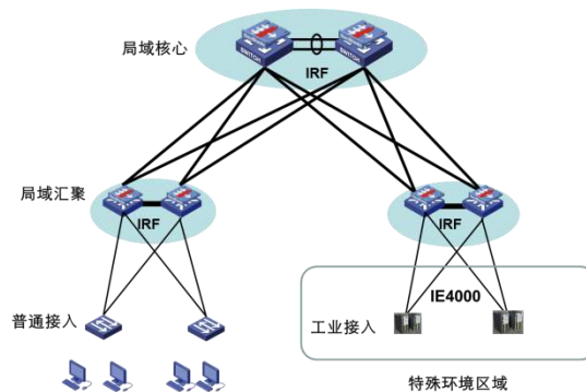
IE4100-LI 系列工业交换机在园区网的应用
