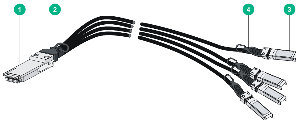
图3-11 QSFP+ to SFP+ DAC 电缆示意图
