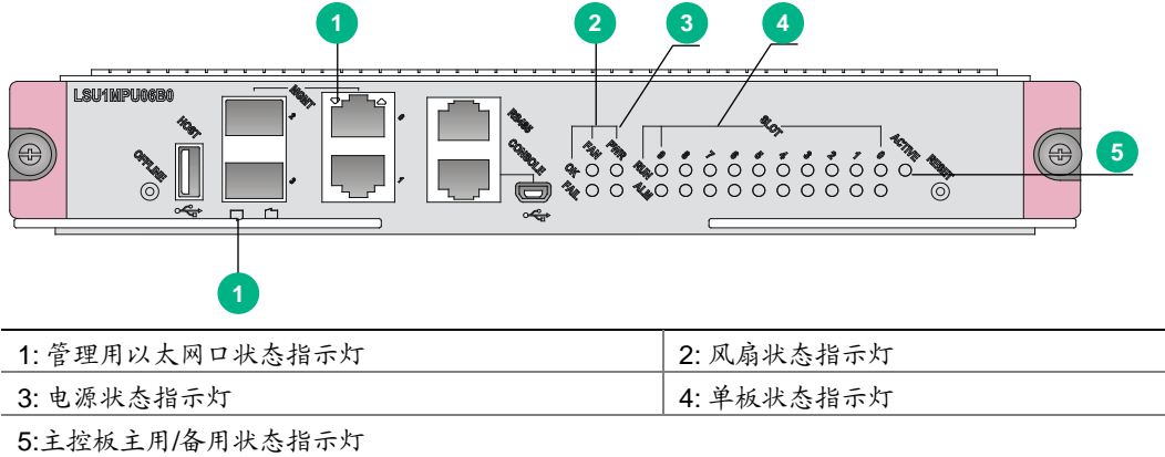
图3-2 LSUM1MPU06B0 主控板指示灯示意图
