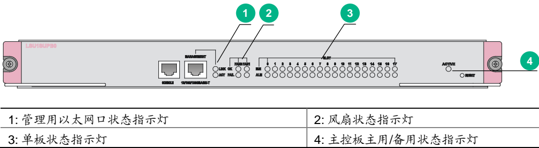
图3-1 LSU1SUPB0 主控板指示灯示意图
