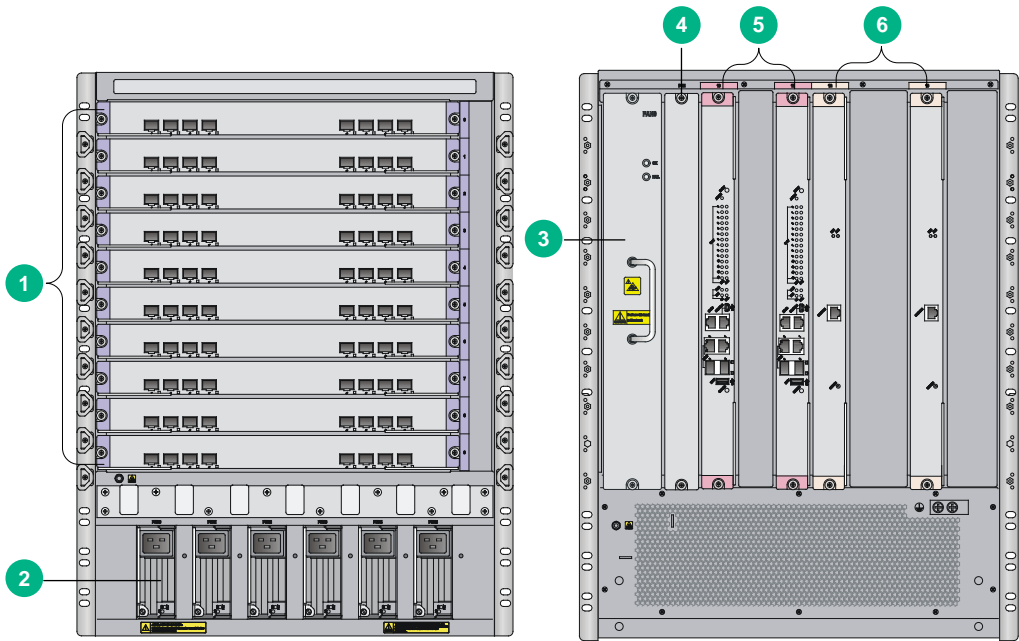
图1-2 S10510 前、后面板示意图
