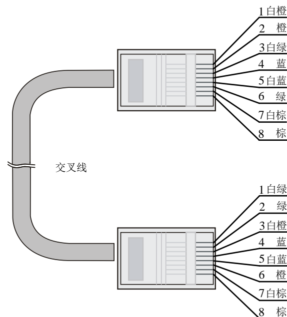
图3-3 交叉线两端线序示意图
