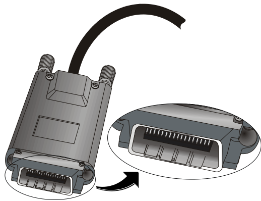
图3-4 InfiniBand 4X 连接器
