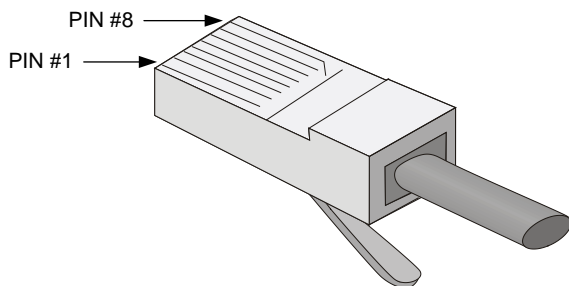
图3-1 RJ-45 连接器引脚序号示意图
