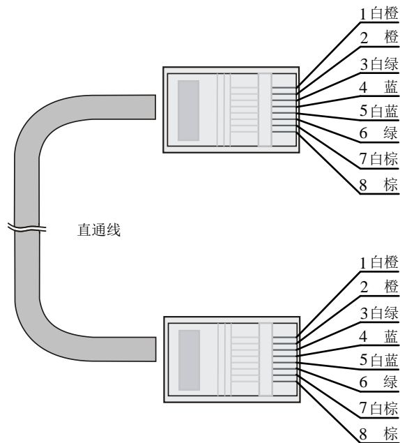
图3-2 直通线两端线序示意图
