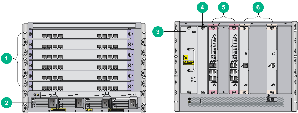
图1-1 S10506 前、后面板示意图
