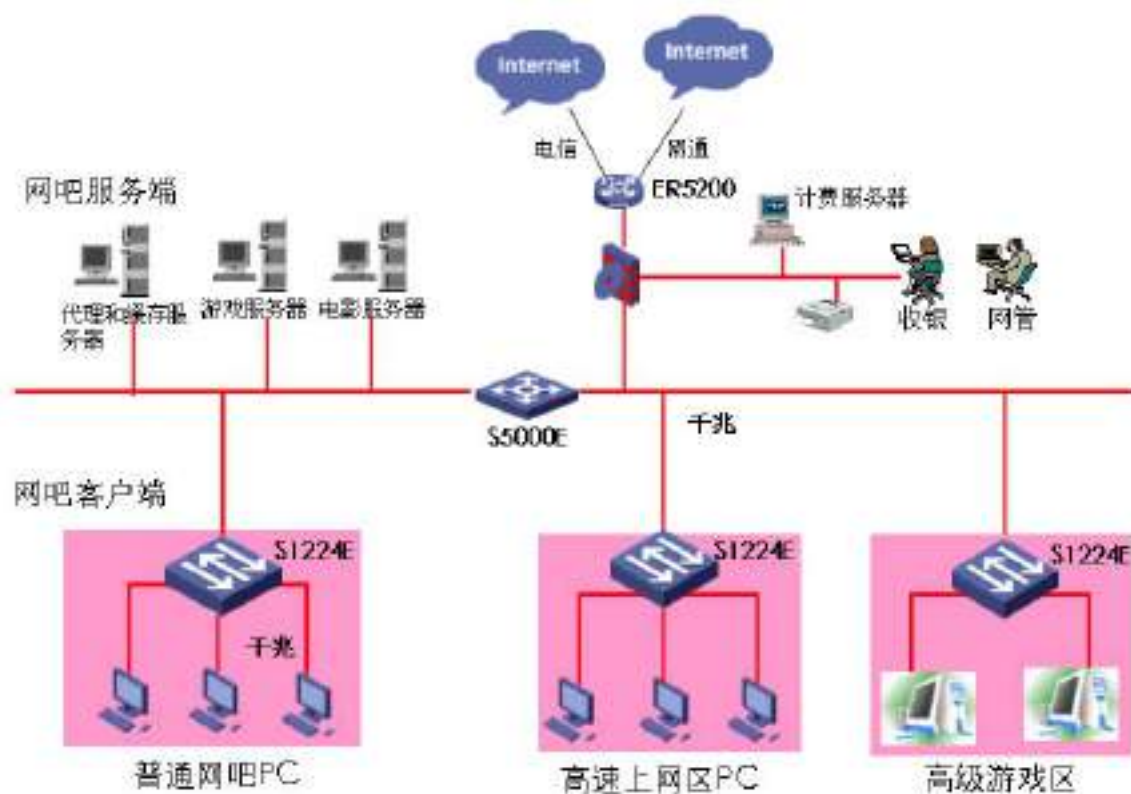
S1224E 以太网交换机千兆网吧应用示意图
