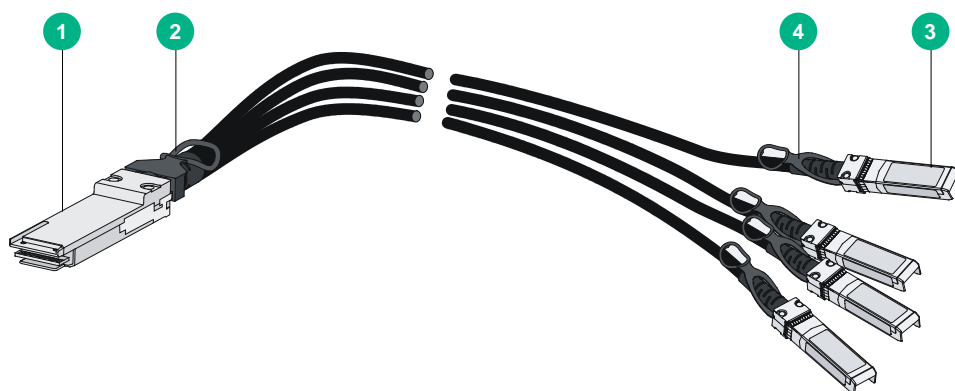
图4-11 QSFP+ to SFP+电缆示意图
