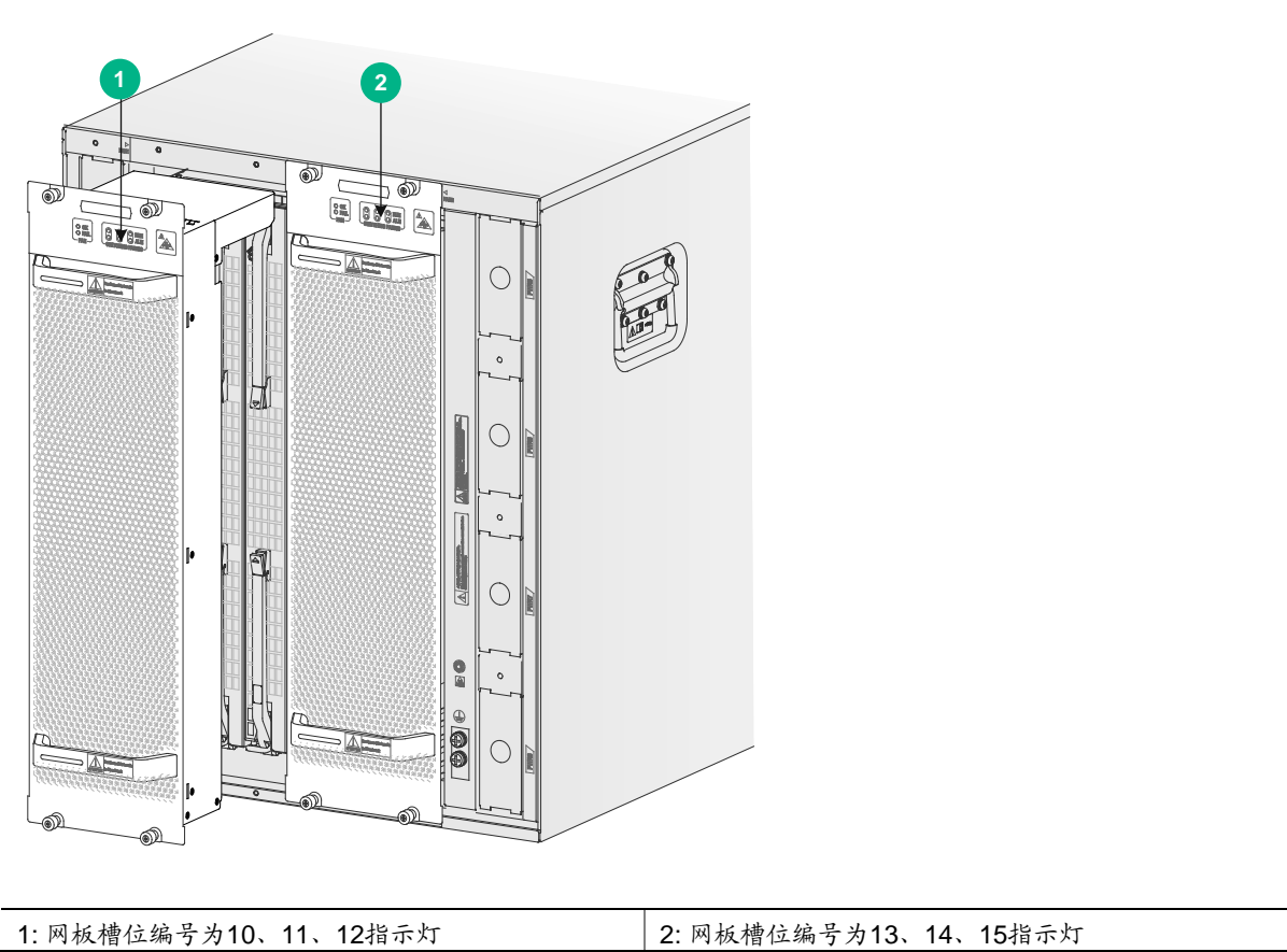
图3-4 风扇框上的网板指示灯与网板槽位对应关系（以 S12508G-AF 为例）
