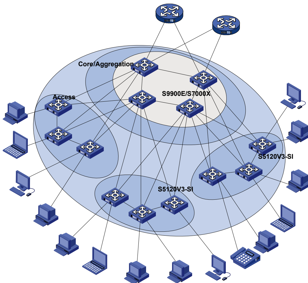
S5120V3-SI接入层组网应用
