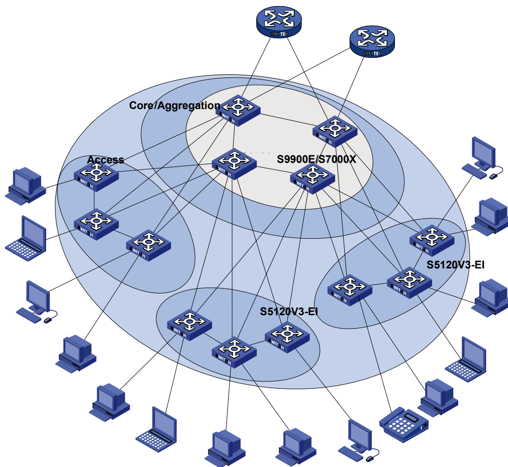
S5120V3-EI接入层组网应用
