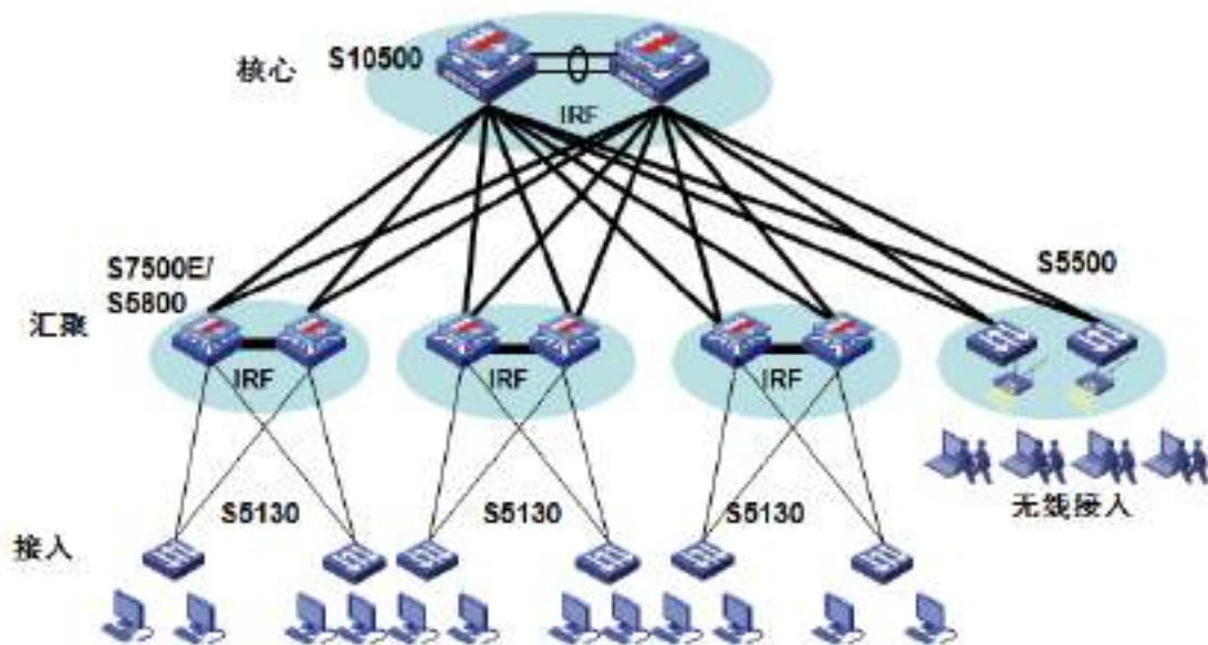
S5130S-MP-EI 系列以太网交换机在企业网/园区网汇聚层应用
