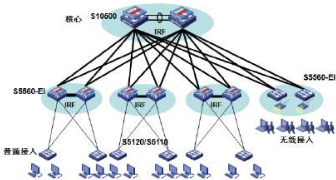
S5560-EI 系列以太网交换机在企业网/园区网汇聚层应用
