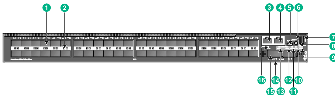
图2-7 S6520X-54HC-EI &amp; S6520X-54HC-HI 前面板示意图
