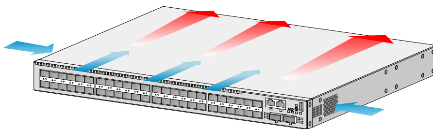
图5-2 交换机散热空气流向示意图二（以 S6520X-30HF-EI 安装 LSPM1FANSA-SN 为例）
