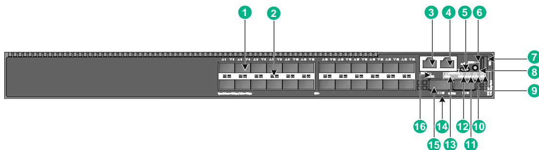
图2-5 S6520X-30HC-EI & S6520X-30HC-HI 前面板示意图
