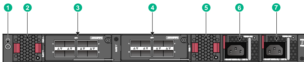
图2-8 S6520X-54HC-EI &amp; S6520X-54HC-HI 后面板示意图
