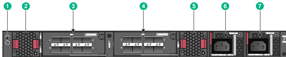
图2-4 S6520X-54QC-EI & S6520X-54QC-HI 后面板示意图
