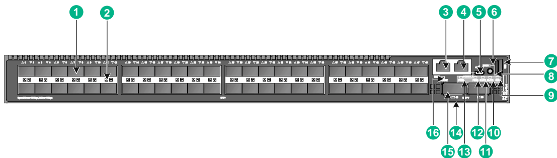
图2-3 S6520X-54QC-EI & S6520X-54QC-HI 前面板示意图
