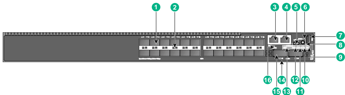
图2-1 S6520X-30QC-EI & S6520X-30QC-HI 前面板示意图
