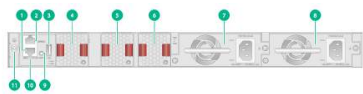
图2-10 S6520X-30HF-EI&amp;S6520X-30HF-HI 后面板示意图
