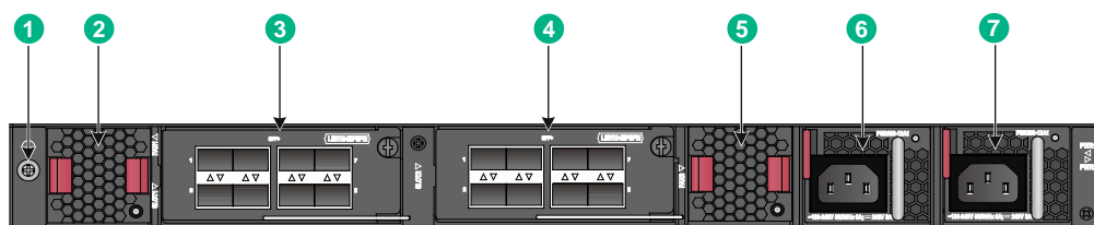
图2-6 S6520X-30HC-EI &amp; S6520X-30HC-HI 后面板示意图
