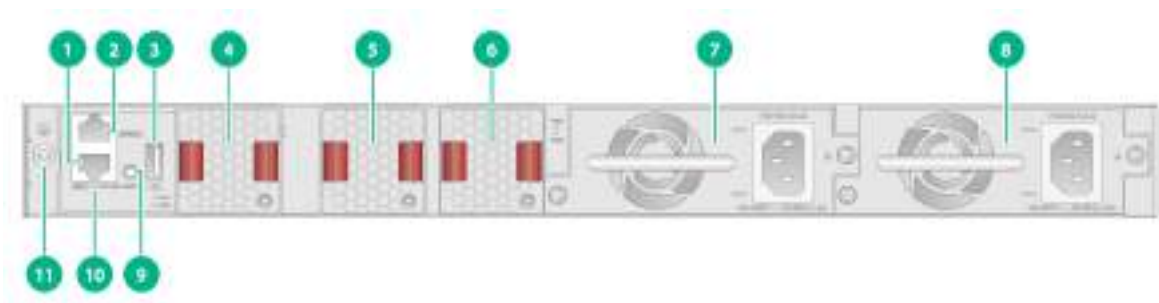
图2-12 S6520X-54HF-EI&amp;S6520X-54HF-HI 后面板示意图
