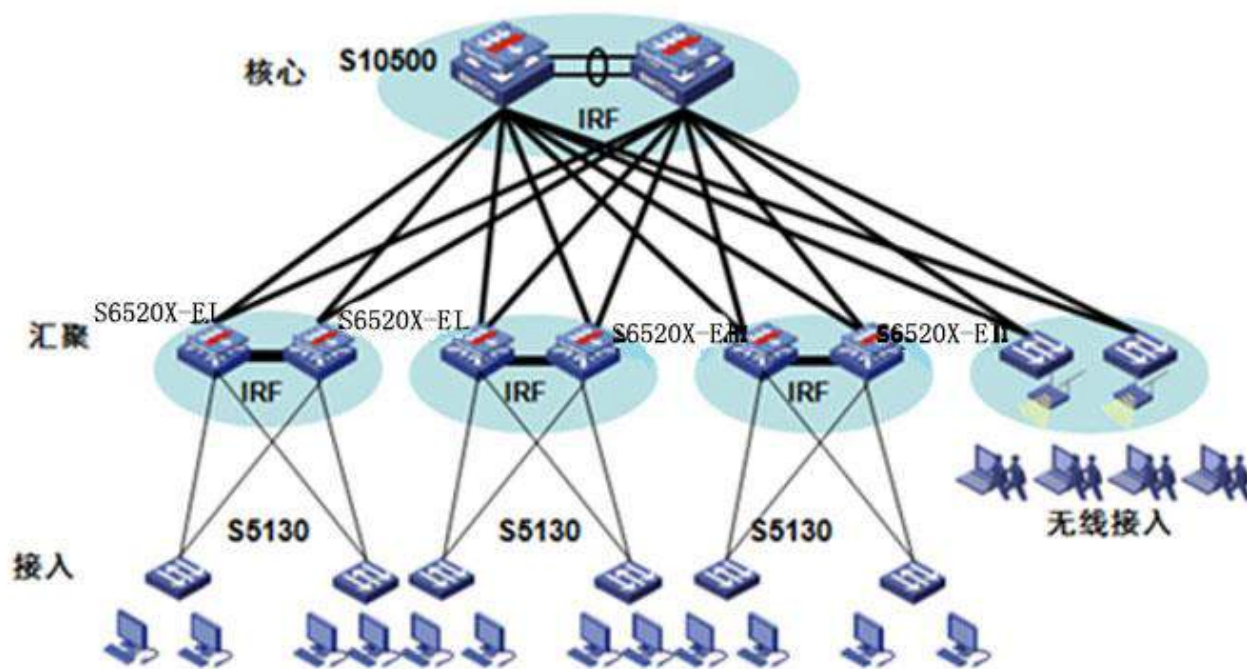
S6520X-EI 系列交换机在园区网的三层组网应用
