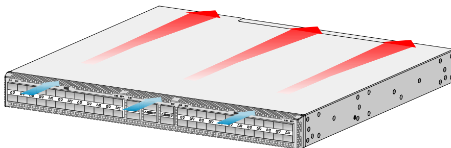
图5-3 端口侧进入电源侧排出散热空气流向示意图（以 S6525XE-54HF-HI 选配 LSPM1FANSB-SN 为例）
