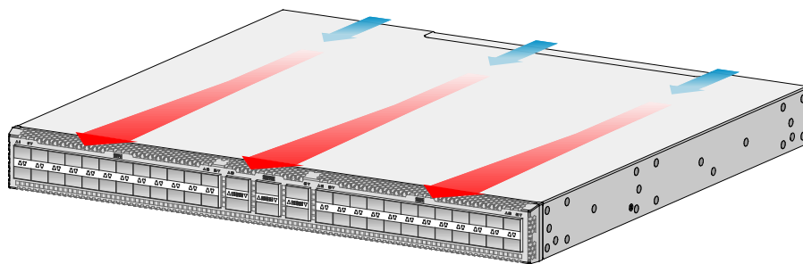
图5-2 电源侧进入端口侧排出散热空气流向示意图（以 S6525XE-54HF-HI 选配 LSPM1FANSA-SN 为例）
