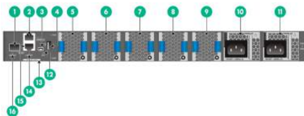
图2-2 S6525XE-54HF-HI 后面板示意图
