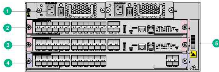
图1-3 S7503E-M 前面板示意图
