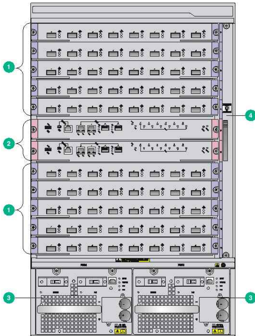
图1-11 S7510E 前面板示意图
