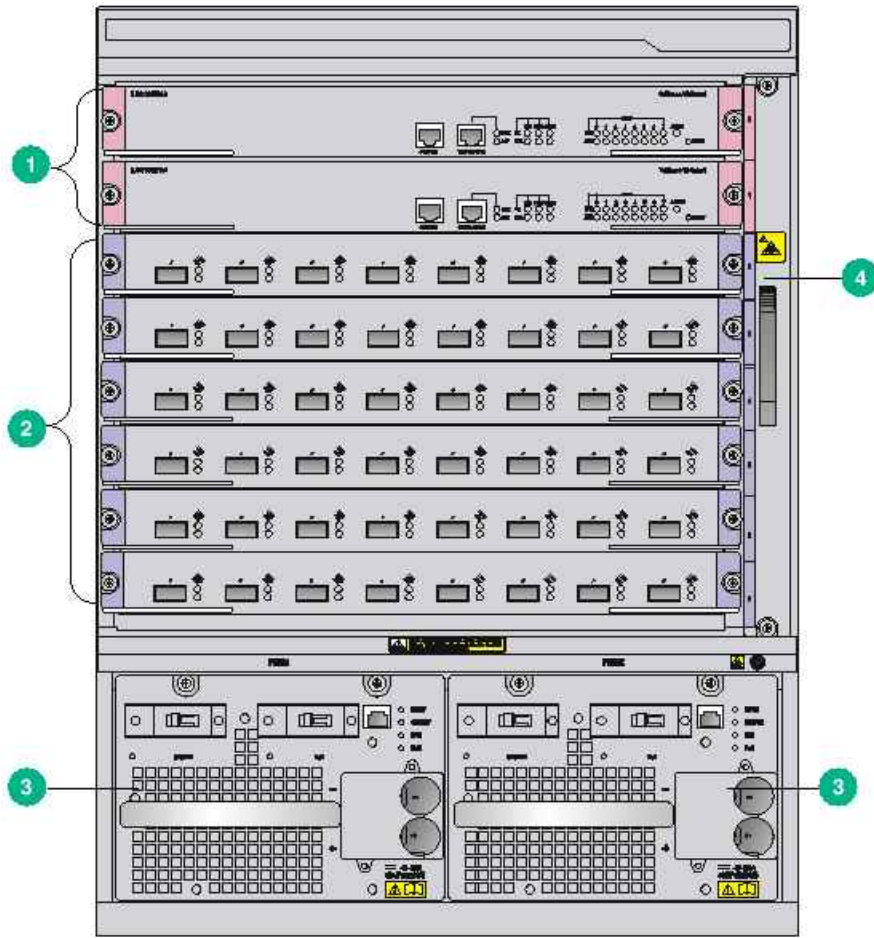
图1-5 S7506E-S 前面板示意图
