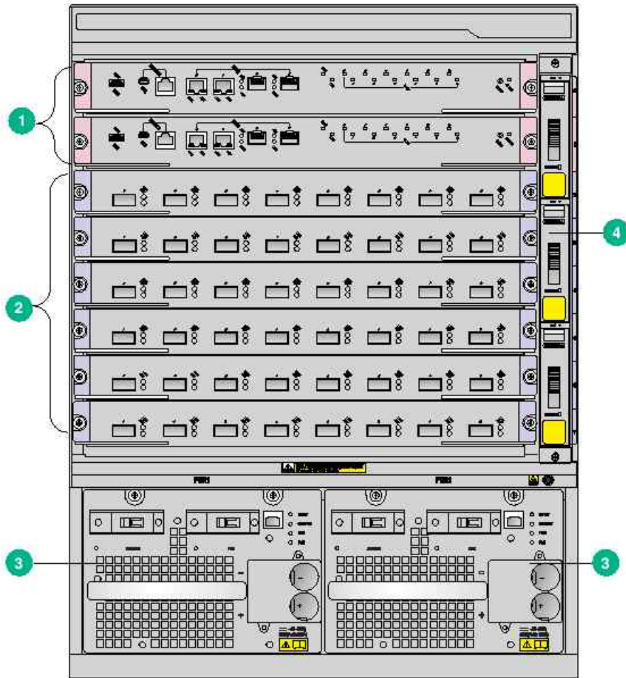
图1-8 S7506E-MF 前面板示意图
