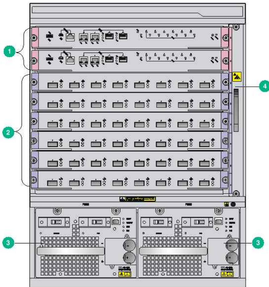
图1-6 S7506E 前面板示意图
