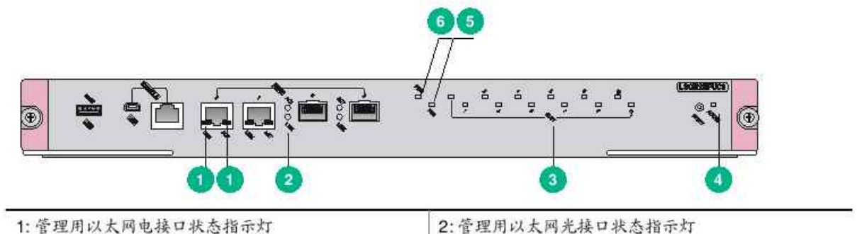
图3-2 主控板指示灯示意图（二）
