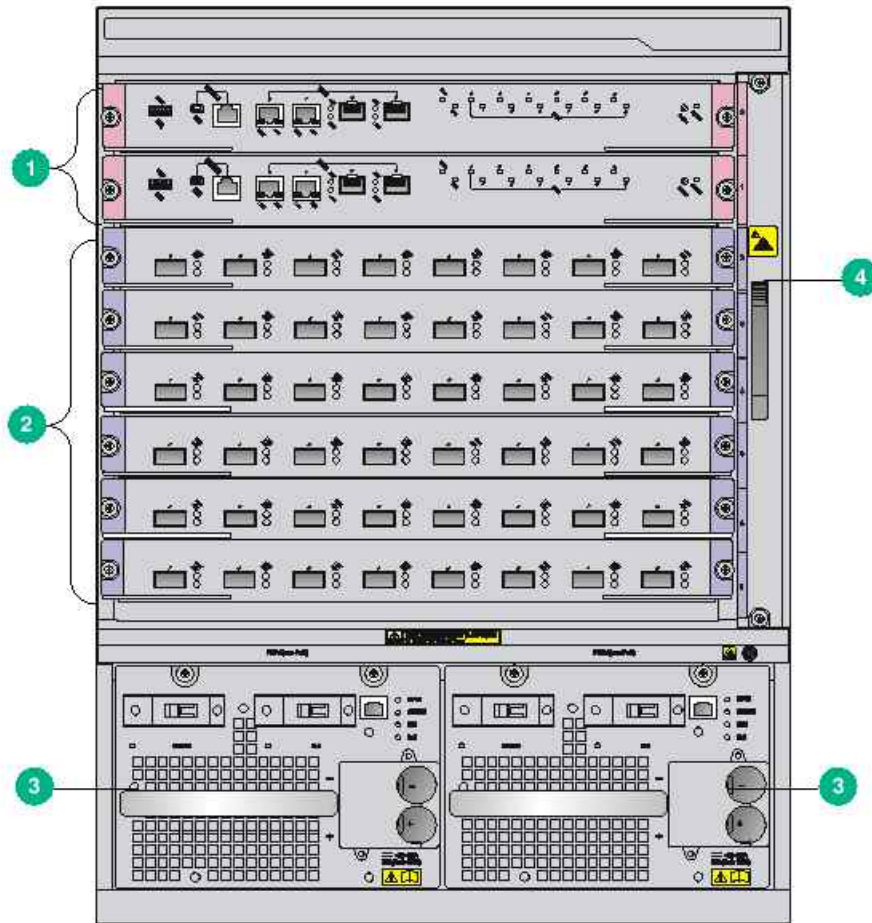
图1-7 S7506E (非 PoE) 前面板示意图
