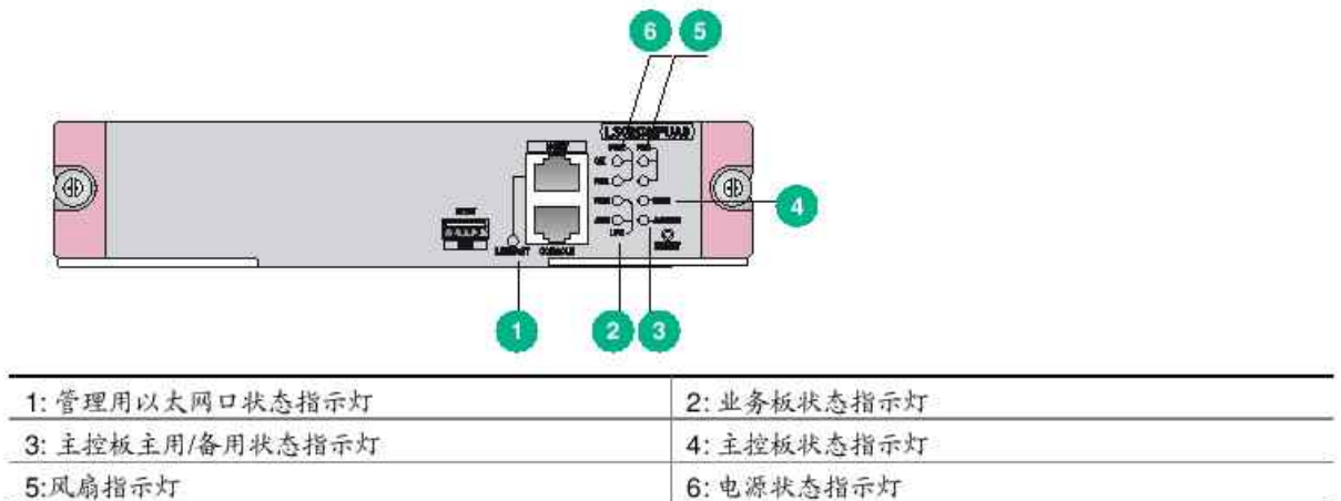
图3-1 主控板指示灯示意图（一）
