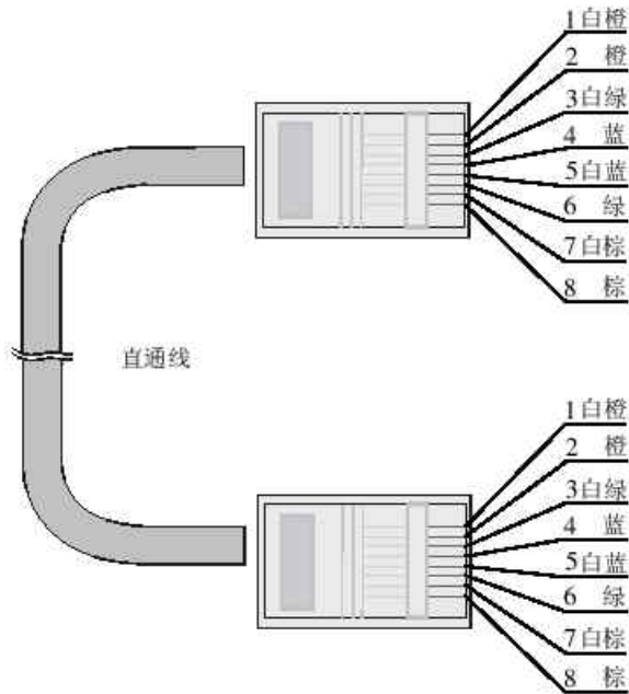
图4-2 直通线两端线序示意图
