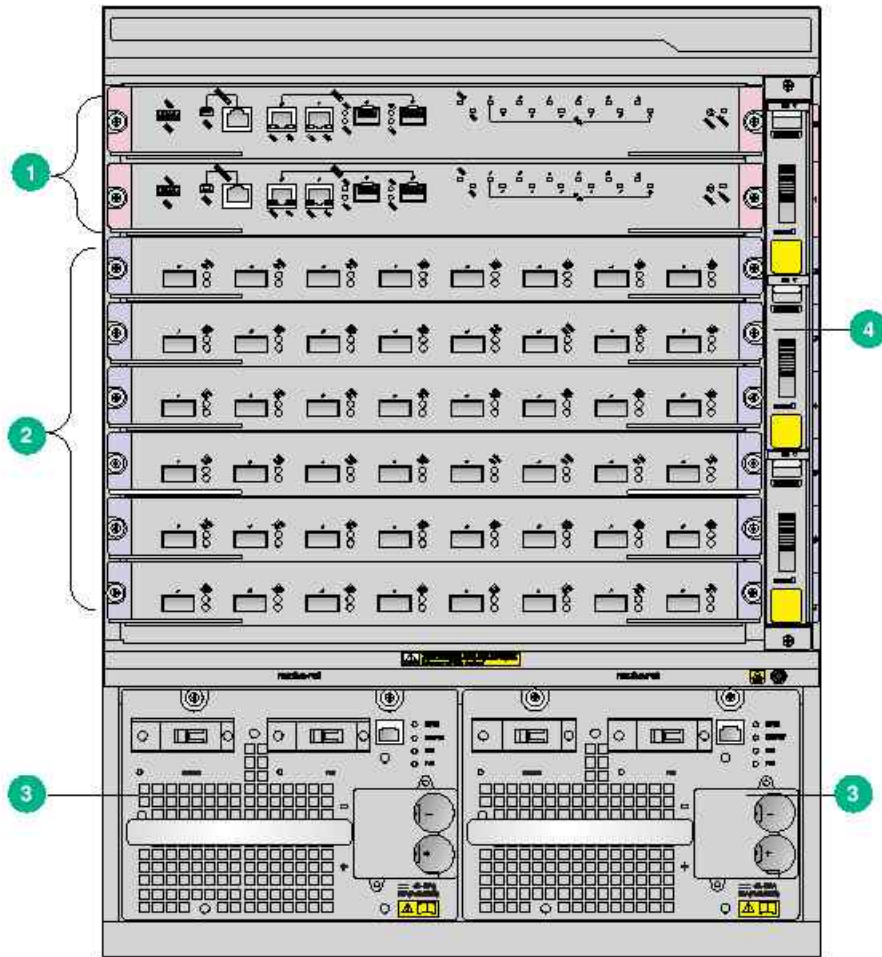
图1-9 S7506E-MF (非 PoE) 前面板示意图
