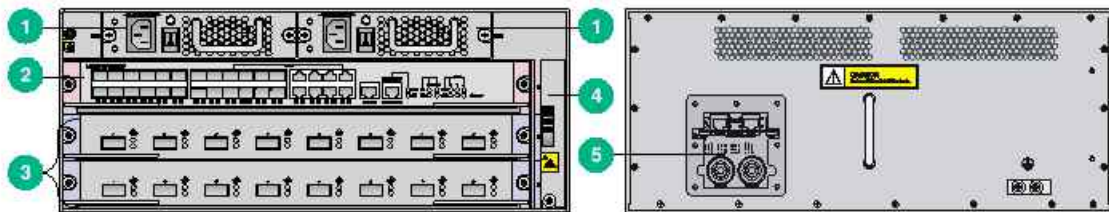
图1-2 S7503E-S 前后面板示意图
