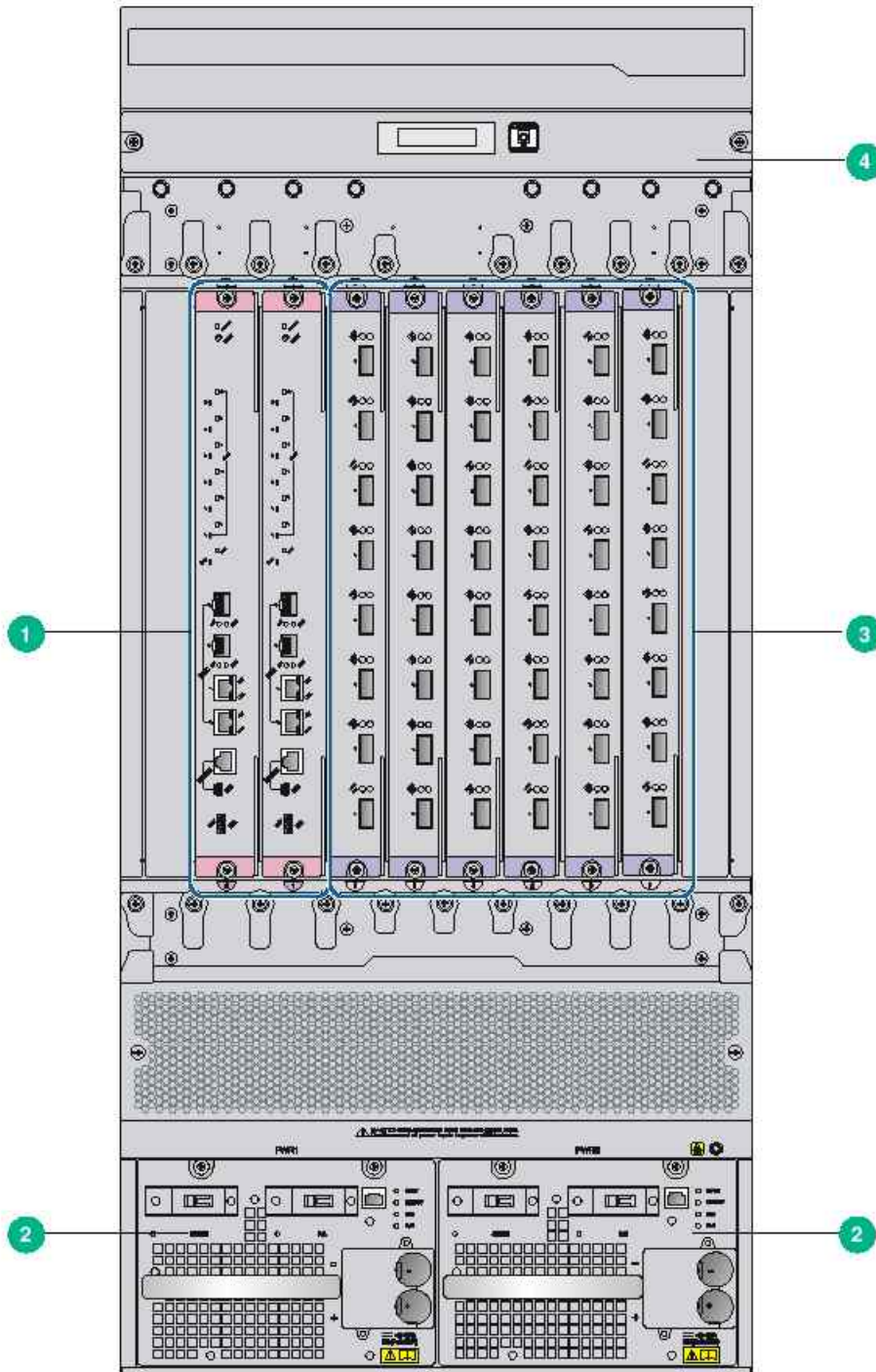
图1-10 S7506E-V 前面板示意图
