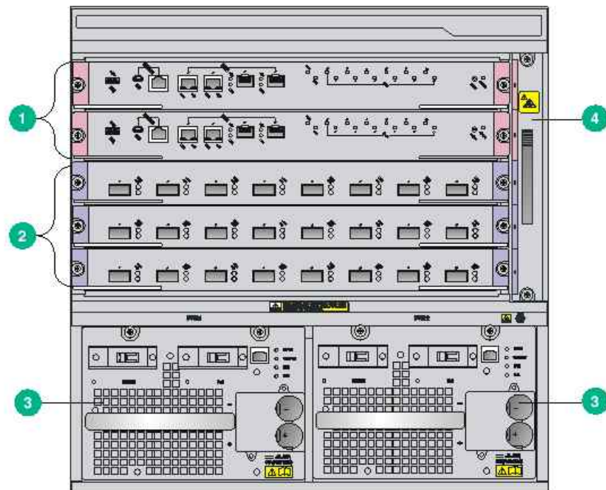
图1-4 S7503E 前面板示意图
