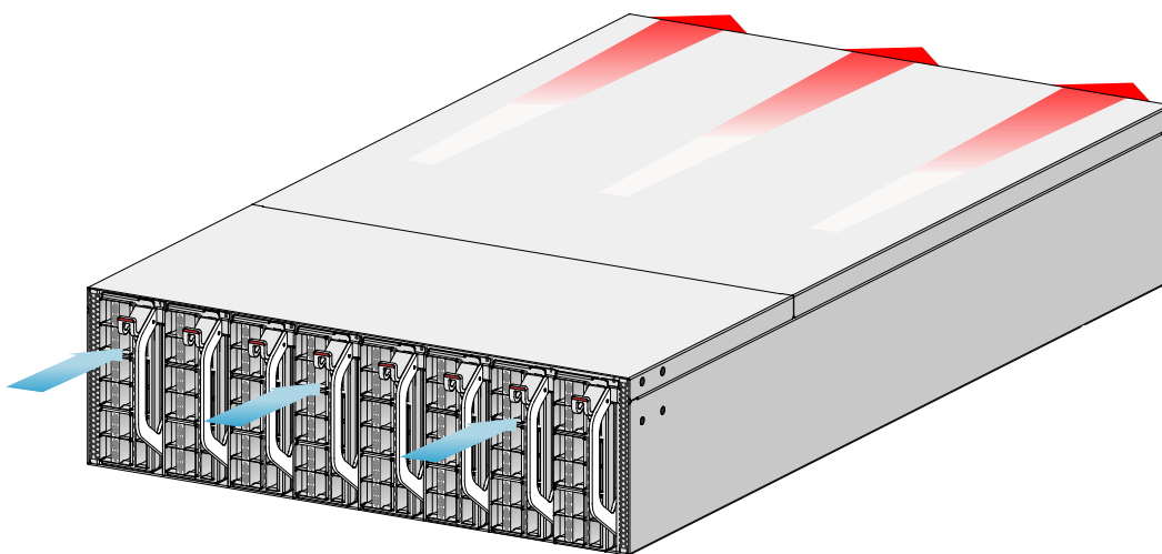
图5-1 端口侧进入电源侧排出散热空气流向示意图（以 S9820-8C 安装 FAN-80B-1-B 为例）
