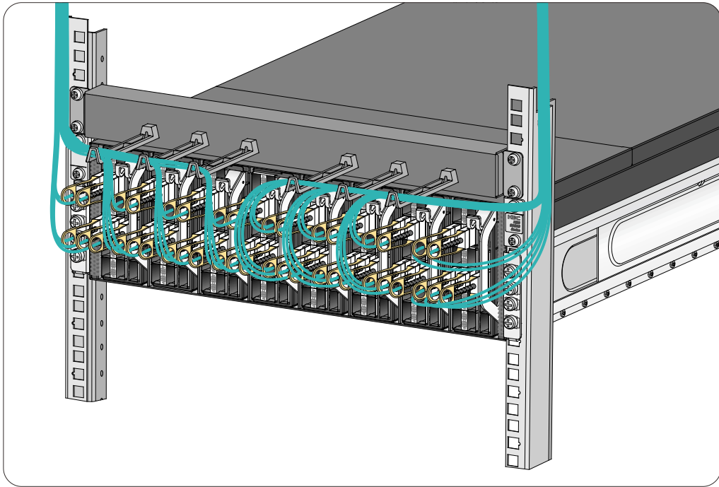
图6-1 S9820-8C 以太网交换机布线示意图
