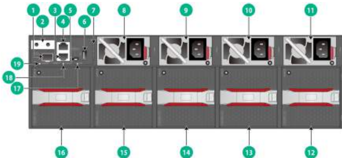
图2-2 S9820-8C 后面板示意图
