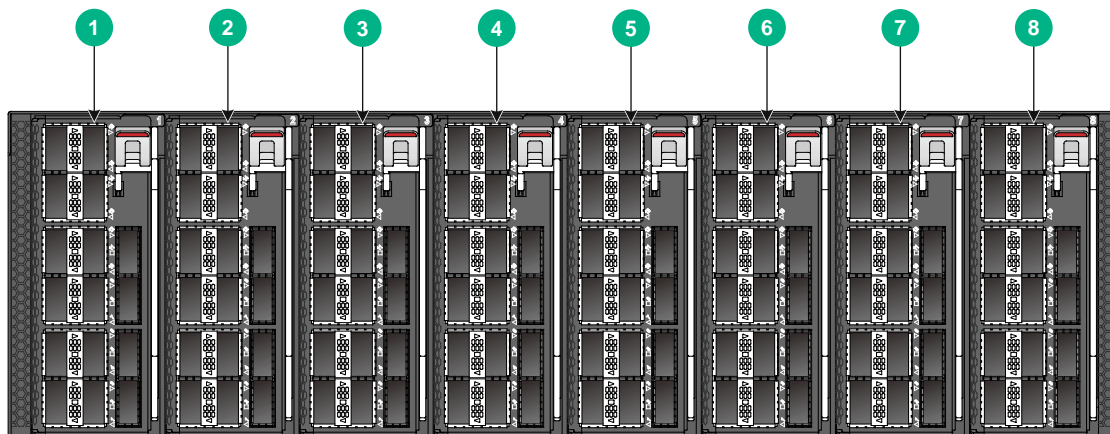
图2-1 S9820-8C 前面板示意图
