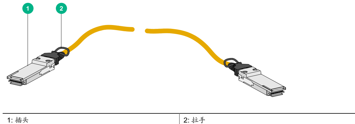
图4-8 QSFP+ AOC 光缆示意图
