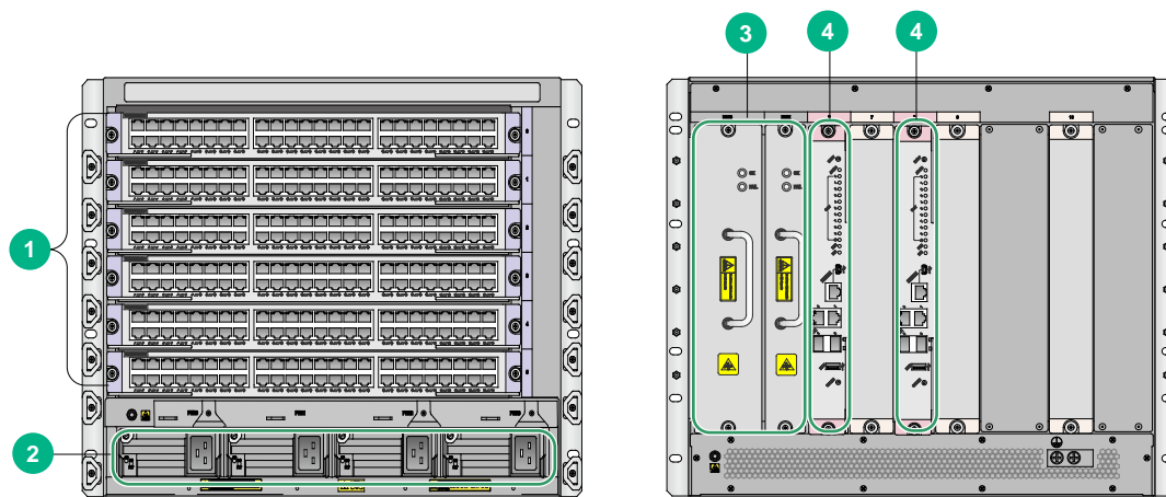
图1-1 S9906X 前、后面板示意图
