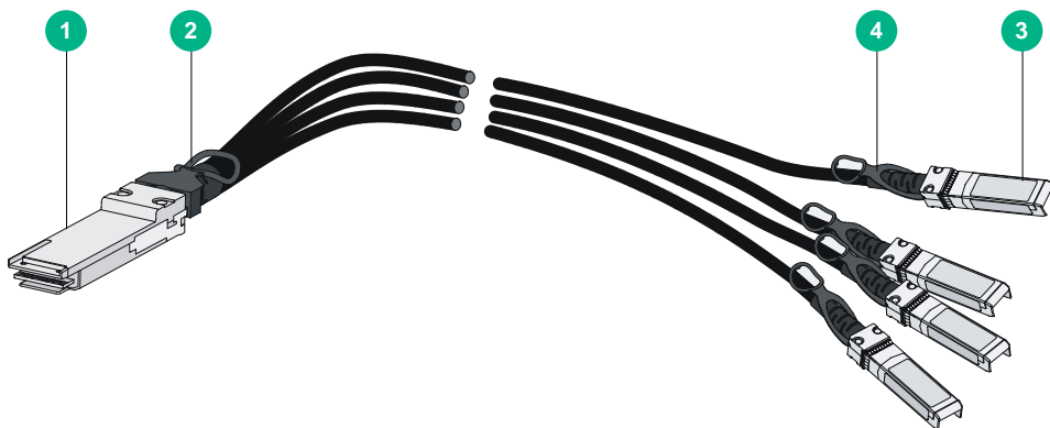
图4-11 QSFP+ to SFP+ DAC 电缆示意图
