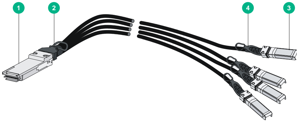
图4-12 QSFP28 to SFP28 DAC 电缆示意图
