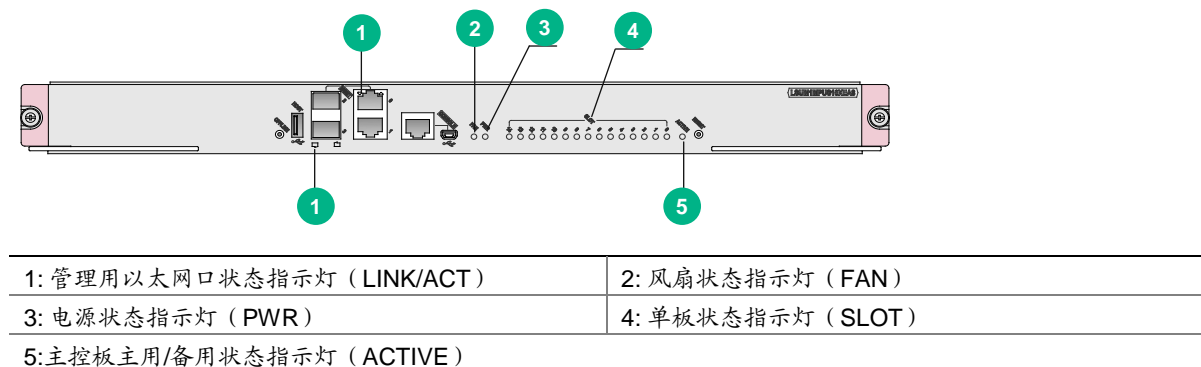
图3-2 LSUM1MPUS10XE8 主控板指示灯示意图
