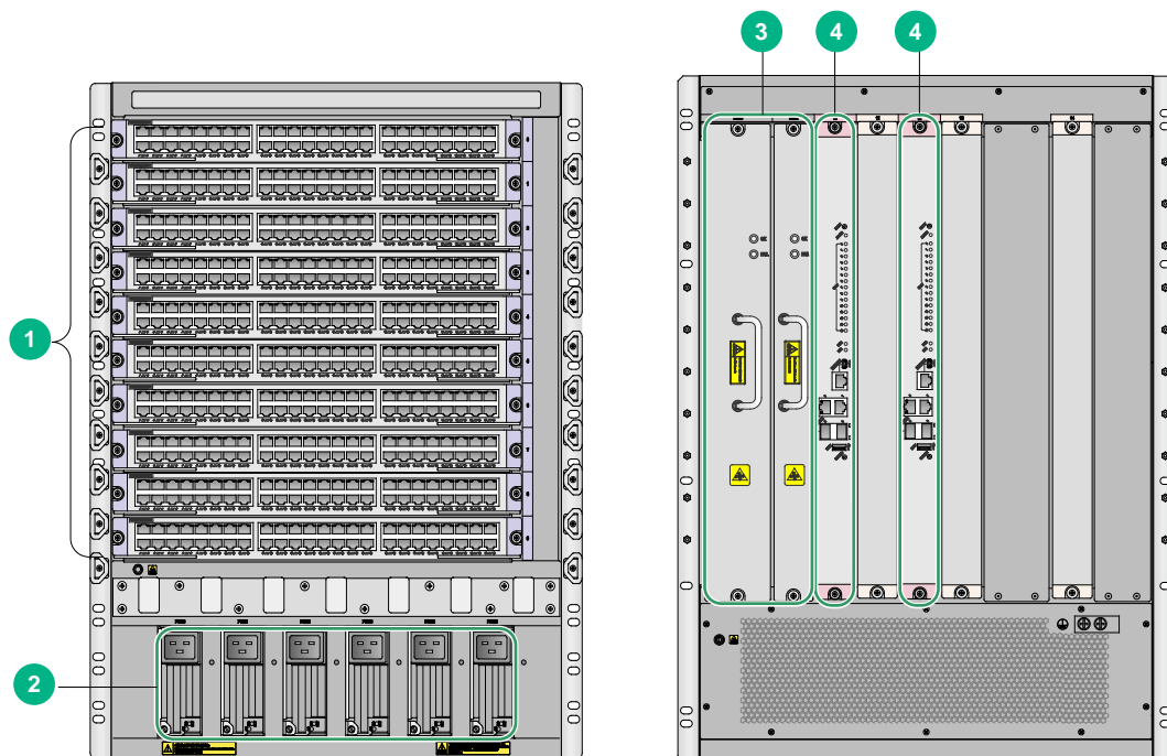
图1-2 S9910X 前、后面板示意图
