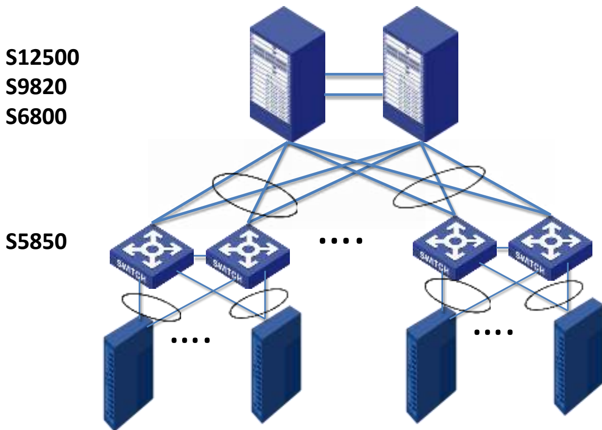
S5850 系列交换机在经典数据中心的接入组网
