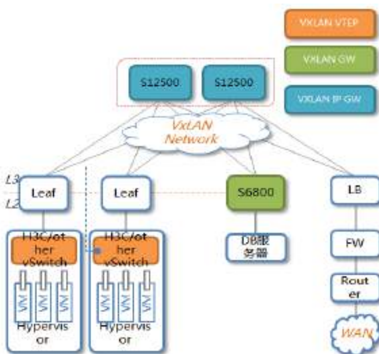
S12500 系列核心交换机 SDN/VxLAN 应用示意图
