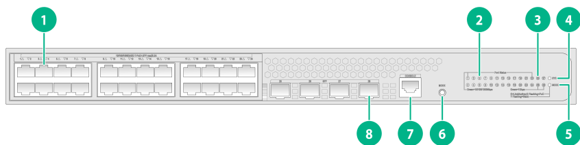
图2-1 US328S-P 前面板示意图
