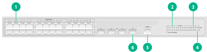
图2-3 US328S 前面板示意图
